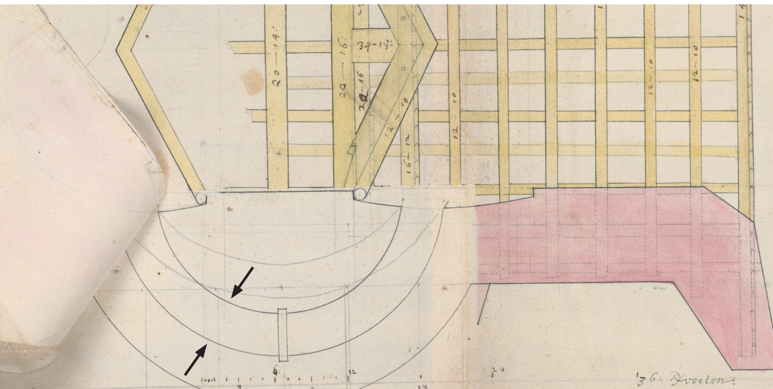
Detail van de plattegrond uit 1701 (zie p. 20). Op bovenstaande tekening is, onder een flap, in inkt, een alternatief verloop van het omloopriool getekend, zie pijlen. Dit verloop komt overeen met het omloopriool zoals boven op de tekening is weergegeven. Klaarblijkelijk waren bij het maken van de bouwtekening de omloopriolen onderwerp van discussie (bron: Nationaal Archief, Plans van Gebouwen, inv.nr. C7).
